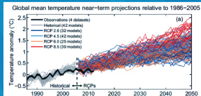
Figure 1. Reproduction de la figure TS.14(a) du rapport AR5 du Giec montrant (i) que les modèles de climat virtuel (en couleur) ne sont pas du tout d'accord entre eux, (ii) qu'ils prévoient des températures plus élevées que les observations (en noir). La figure 2, ci-dessous, montre que la «pause» observée depuis 1998 se prolonge aux fluctuations près.
