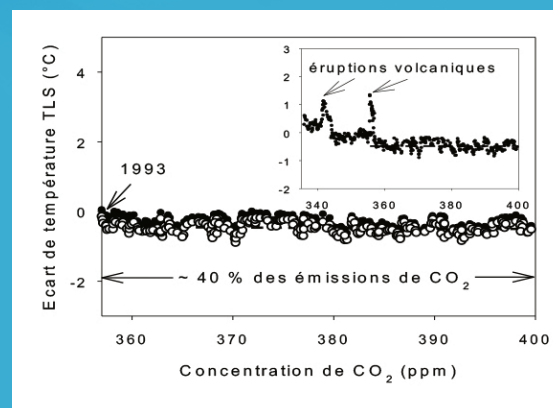
Figure 3. Absence d'évolution de la température mesurée dans la basse stratosphère (à ~ 17 km d'altitude) par les satellites RSS (o) et UAH (●) dans une période correspondant pourtant à ~ 40 % du CO 2 émis depuis le début de l'ère industrielle, à une altitude où les modèles convectifs de climat prévoient une signature maximale de l'effet de serre atmosphérique.
