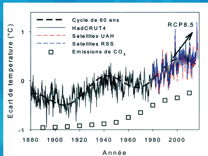
Figure 2. Évolution de la température moyenne de la Terre selon plusieurs sources. Les émissions de CO 2 ne se corrélient évidemment pas à l'oscillation de ~ 60 ans observée. La flèche RCP8.5 pointe vers la température à la fin du siècle prévue par le scénario du Giec sans limitation des émissions, confirmant l'écart grandissant entre mesures et modèles.
